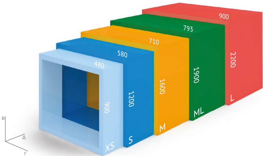
Габариты модулей
